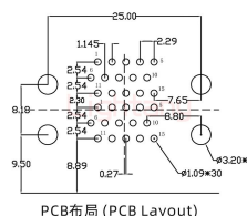
PCB布局 (PCB Layout)
